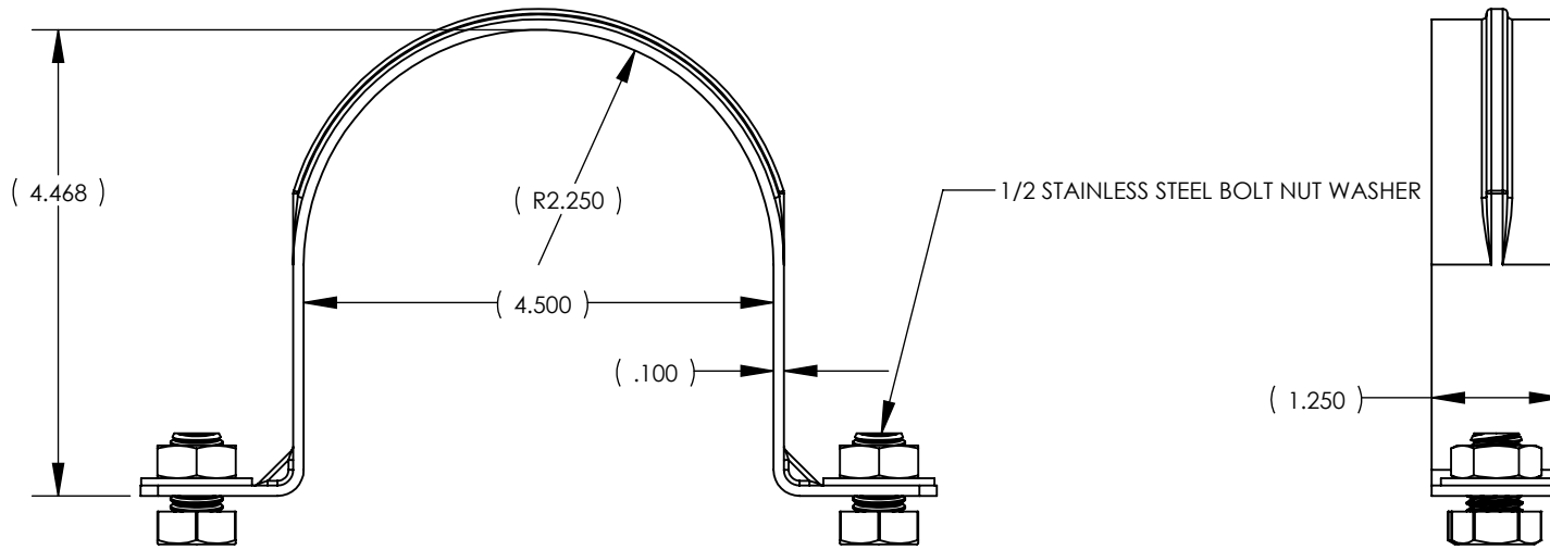
Part No. W-NW-4X00 2 Hole Conduit Strap Aluminum for 4" Conduit
